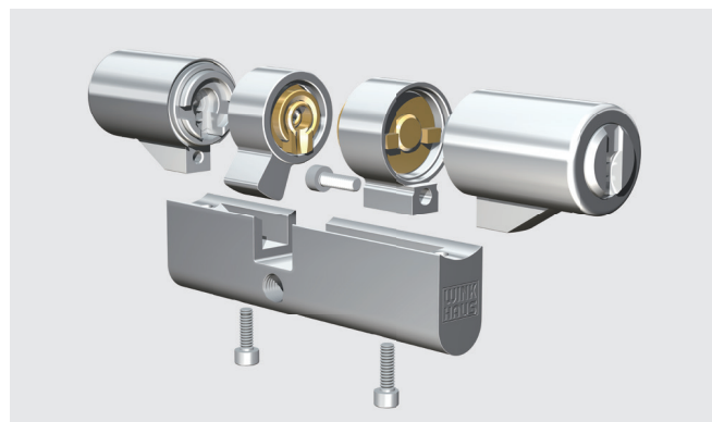
Modułowa budowa wkładki keyTec X-tra umożliwia przebudowę i dopasowanie do drzwi o innej grubości.
